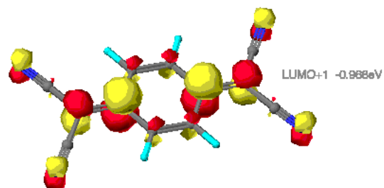
TCNQ
