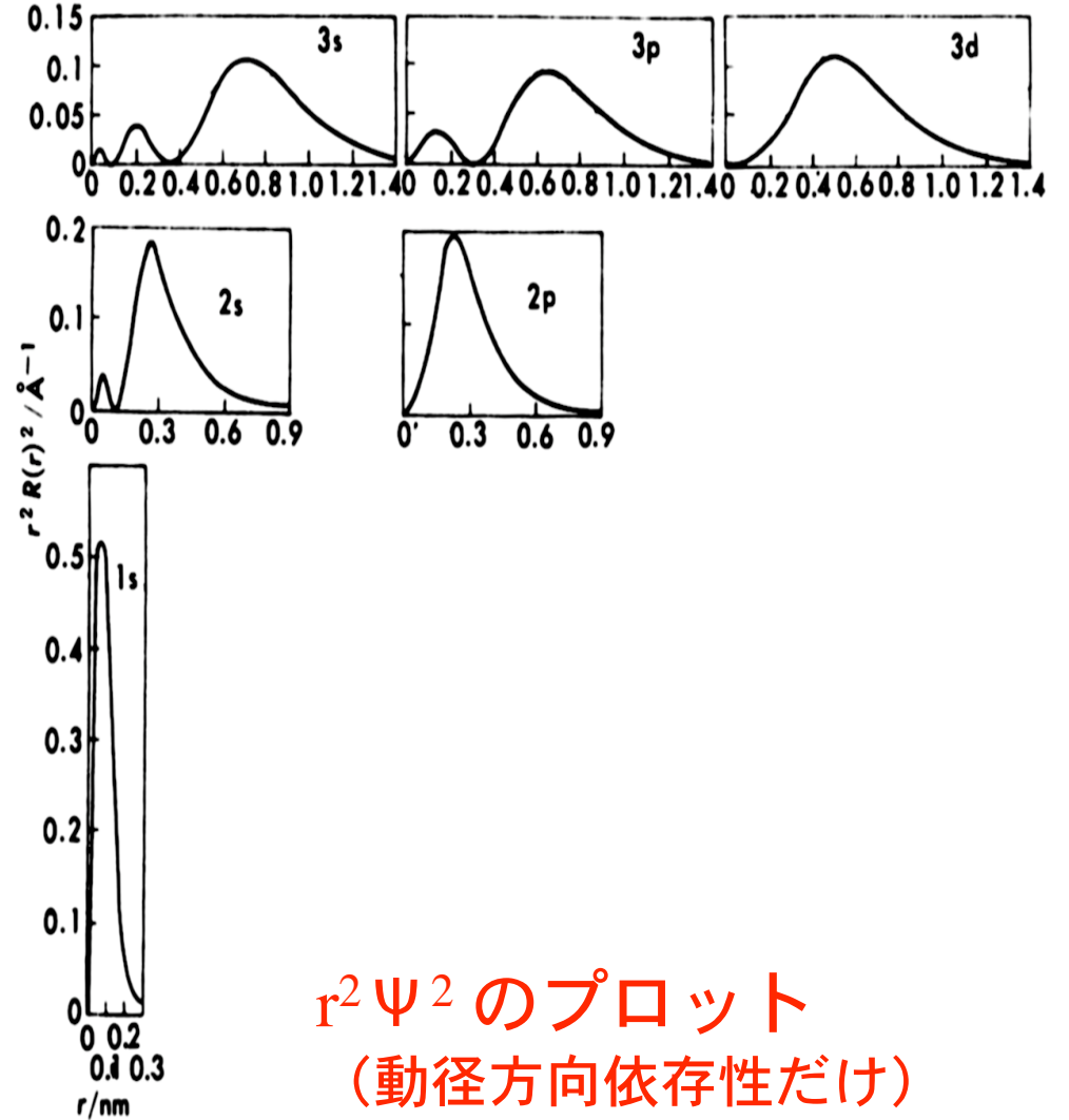
図 11・6 水素原子軌道の動径分布関数 r^2R^2(r)
