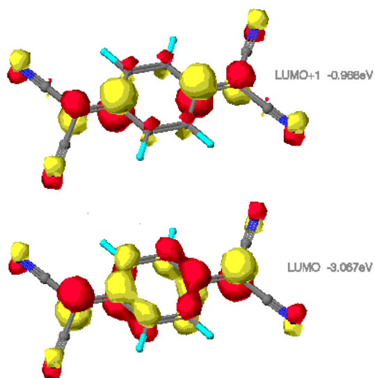
TCNQ
