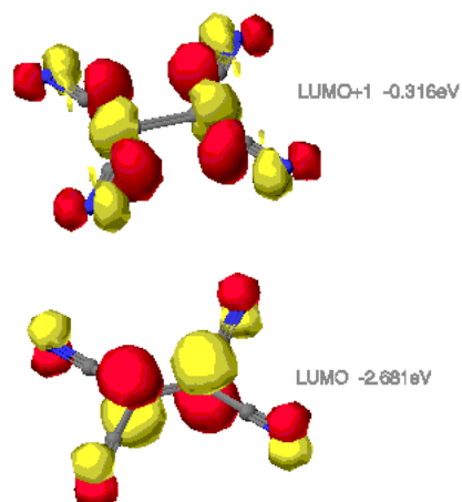
TCNE
