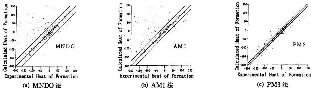
図3 生成熱の計算値と実験値との比較。斜めの直線の両側に標準偏差の誤差幅をつけた。
