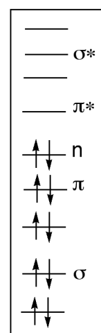
図2 分子軌道準位の一例
