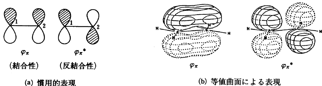
図1 エチレンの \pi , \pi^* 軌道
