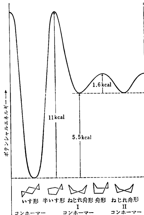
図 9・5 シクロヘキサンのコンホーメーション間のポテンシャルエネルギー関係
