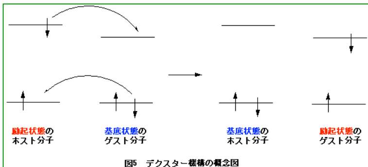
図5 デクスター機構の概念図
