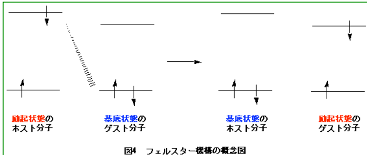
図4 フェルスター機構の概念図
