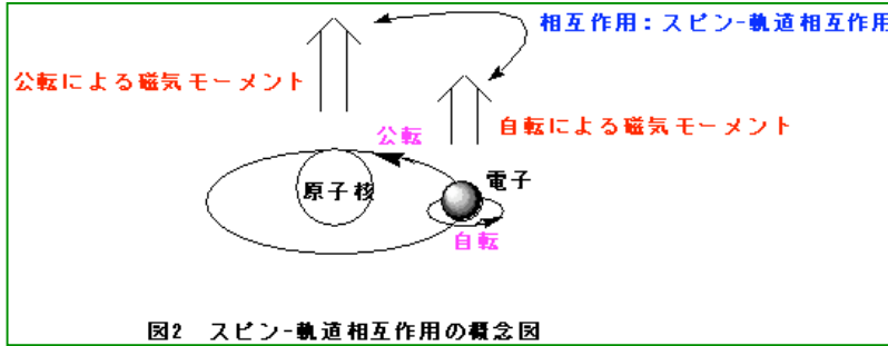
図2 スピン-軌道相互作用の概念図
