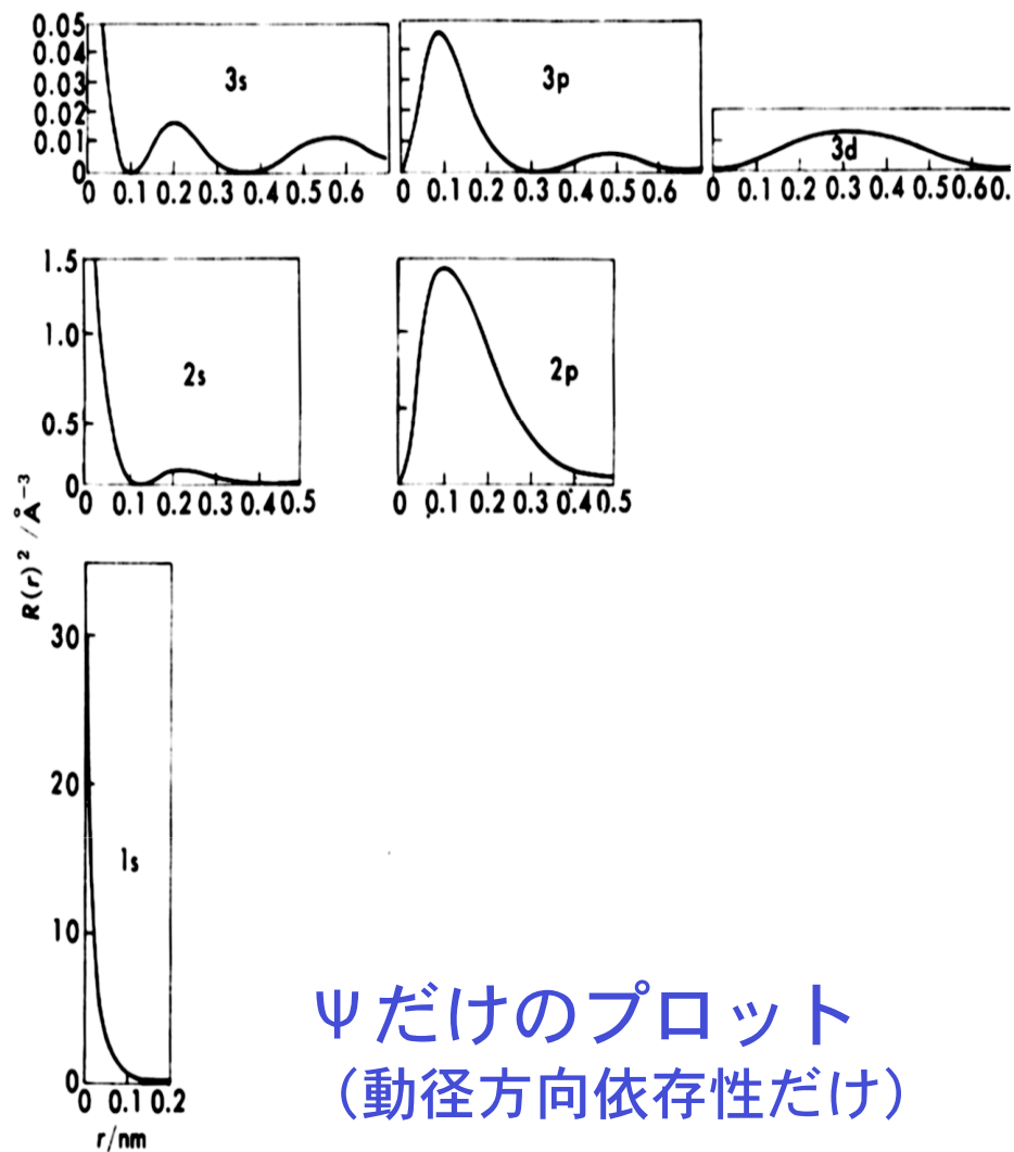
図11・5 水素原子の n=1, 2, 3 の状態の波動関数の動径部分の二乗
