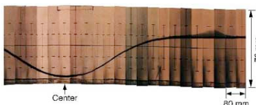
水 (反磁性)
