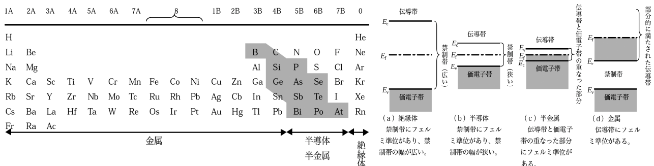
元素周期表と単元素物質の電気的特性
