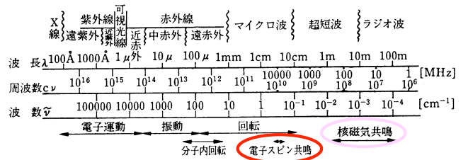
図 1.1 分子による電磁波の吸収
