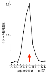
図 6.4 スルメ中のラジカルの濃度分布
