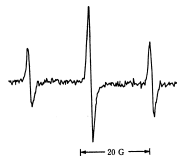
図 1.19 等価な2個の 1 H核による超微細構造
