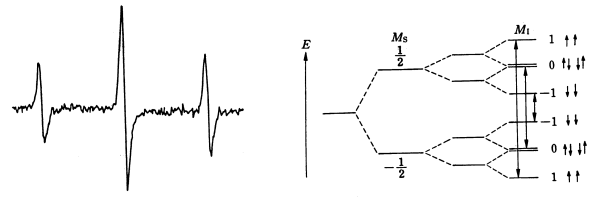
図 1.19 等価な2個の ^1H 核による超微細構造 図 1.20 等価な2個の ^1H 核による超微細相互作用
