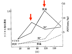
図 6.11 ポテトチップス試料中のラジカル量と POV の経日変化
