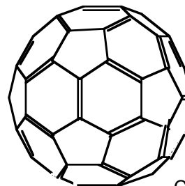
C60
