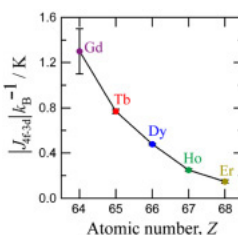
希土類-有機物-遷移金属複合 ナノ磁石の交換相互作用
