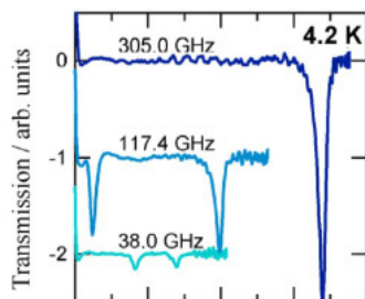
希土類ナノ磁石 [Dy_2Cu_2]_n の 4.2 Kにおける高周波EPRスペクトル
